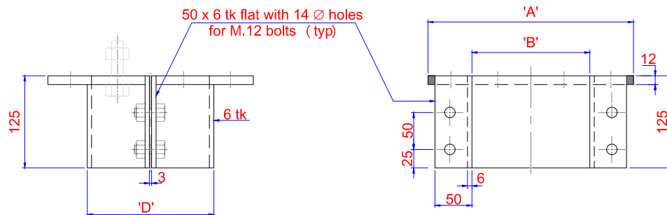
ELEVATION
