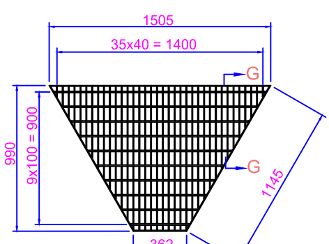
GRATING DETAIL G2 : 5 Nos.
